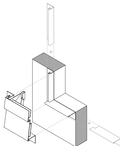
PERSPECTIVE DE L'ASSEMBLAGE DE LA BASE
