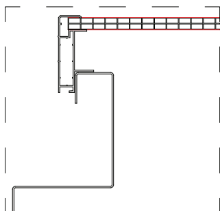
DÉTAIL 01
