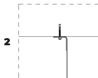
DÉTAIL D'ANCRAGE EN ACIER BÉTON
