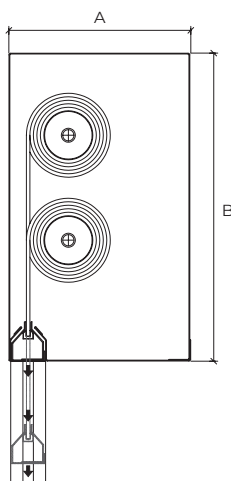
MULTI ENROULEURS CONFIGURATION VERTICALE A: 190-270 mm B: 300-500 mm
