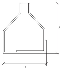
ACIER GALVANISÉ A: 55 mm B: 47 mm
