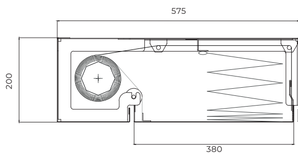
DÉTAIL DE CAISSON BARRIÈRE ÉLEVÉE
