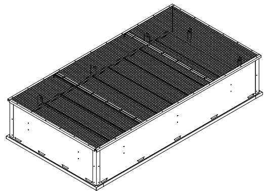
VUE PERSPECTIVE
