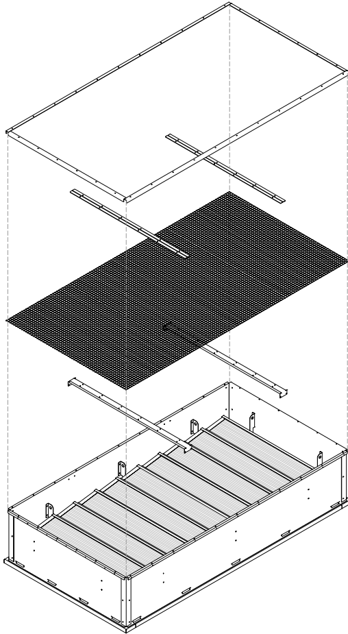
ASSEMBLAGE
